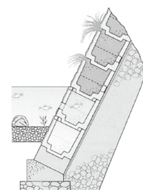
環境保全型ブロックの構造
